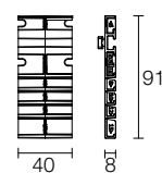
CSP0241-06 Distanziale zoccolo Plinth spacer
